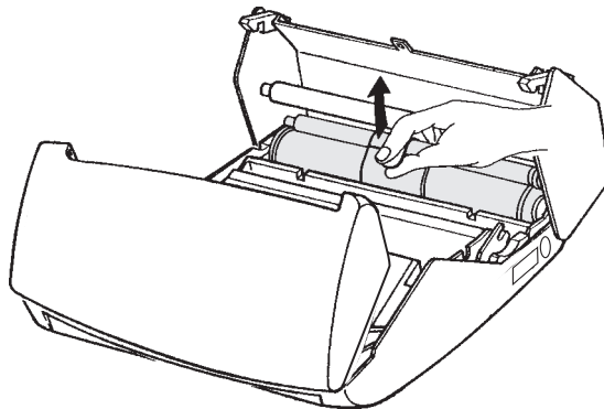
Afbeelding 24: Plakstrip verwijderen.
