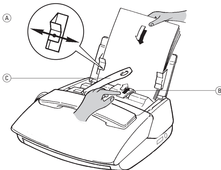
Afbeelding 5: Afdrudpapier plaatsen, invoerknop indrukken en achtergeleider documenten uitschuiven.
