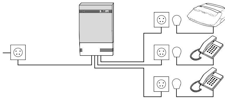
Afbeelding 18: Aansluiten op huis- of bedrijfscentrale.
