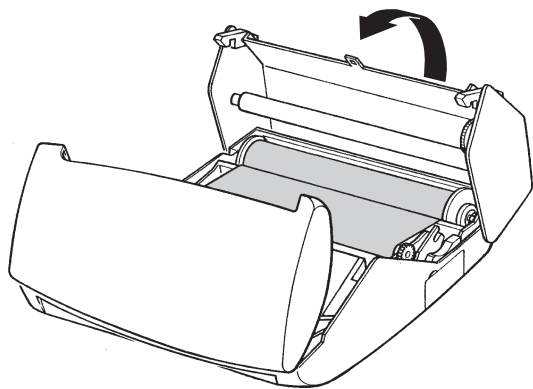
Afbeelding 32: Achterkant fax sluiten.
