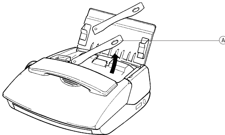
Afbeelding 14: Achtergeleider documentinvoer uitschuiven
