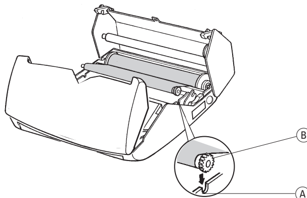
Afbeelding 25: Kleine spoel afdrukrol plaatsen.
