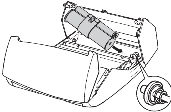
Afbeelding 23: Grote spoel afdrukrol plaatsen.
